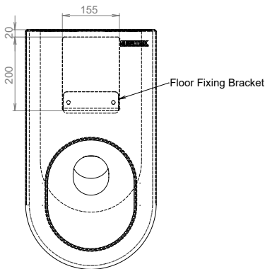
MODEL PCAMS / PCAMP Plan
