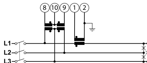
Connessione da 1 TA e 2 TV
