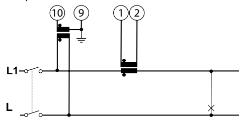
Connessione da 1 TA e 1 TV
