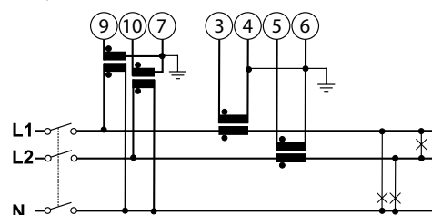
Connessione da 2 CT e 2 VT/PT
