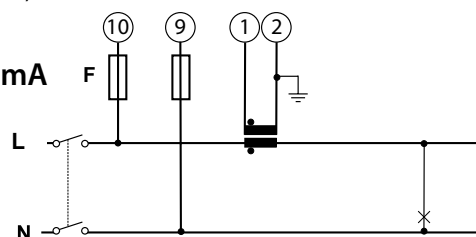
Connessione da 1 TA
