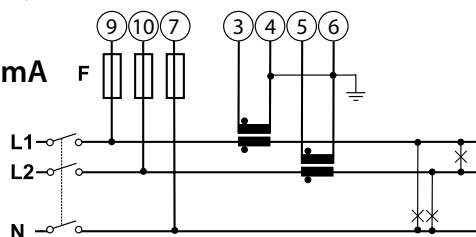
Connessione da 2 TA
