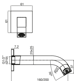
Bloc Bath Outlet
