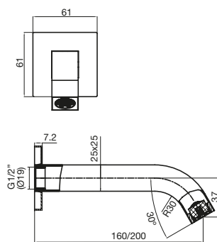
Bloc Bath Outlet
