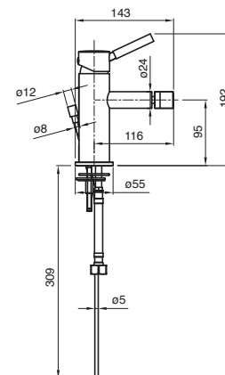
Drift Bidet Mixer
