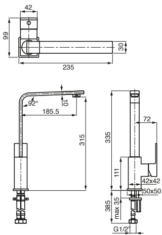
Bloc Sink Mixer
