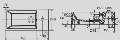
Solus Mini Wall Basin 485mm
