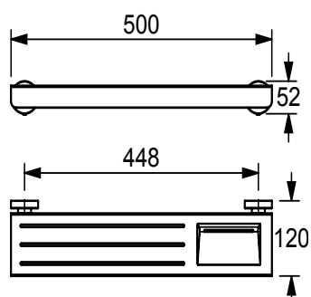
Shelf (Metal)
