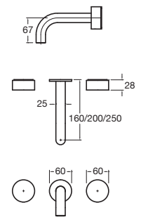
Pure Bath Set
