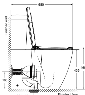
S-Trap
