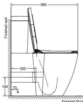
P-Trap
